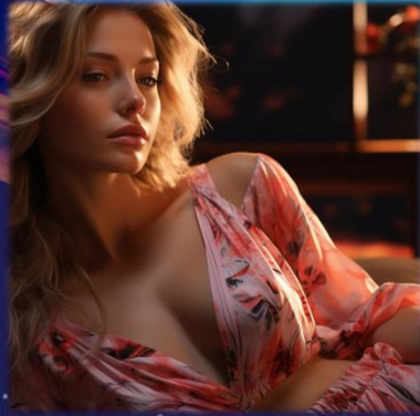
3.AIGC Model
